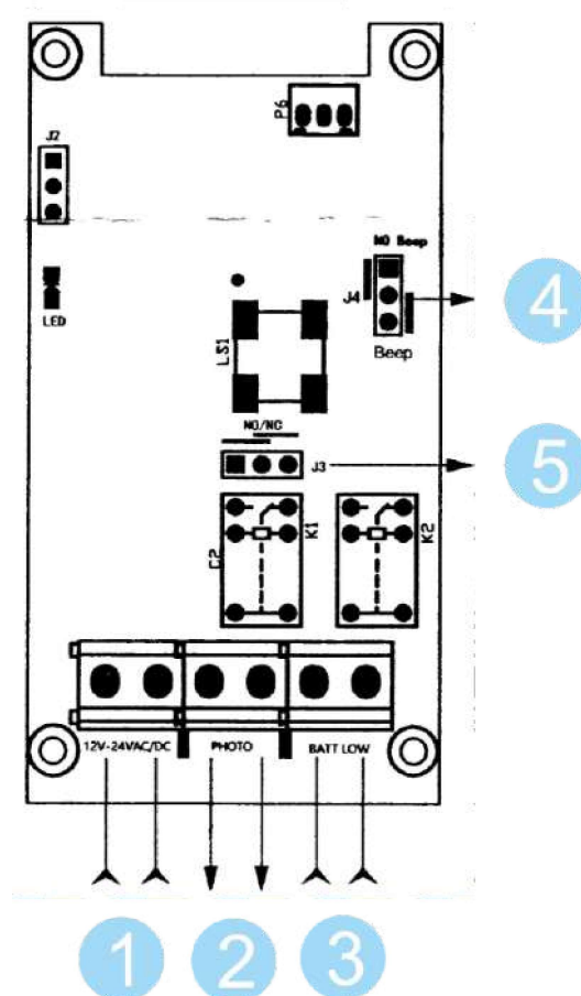
Рисунок 6.9.1.6 Устройство платы приемника
