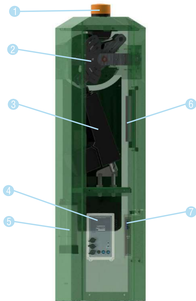
Рисунок 6.1 Внешний вид и состав шлагбаума
