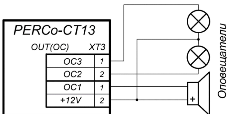
Рисунок 25. Схема подключений дополнительного оборудования к выходам контроллера типа «Открытый коллектор»
