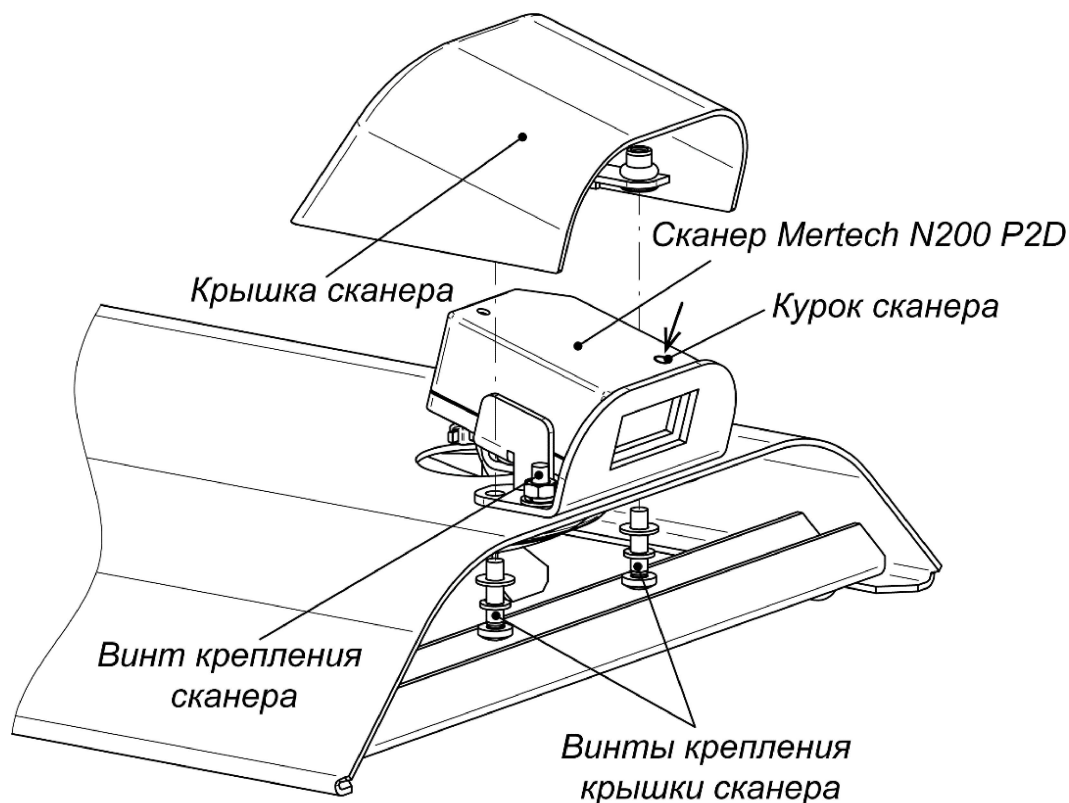
Рисунок 6. Снятие крышки сканера
