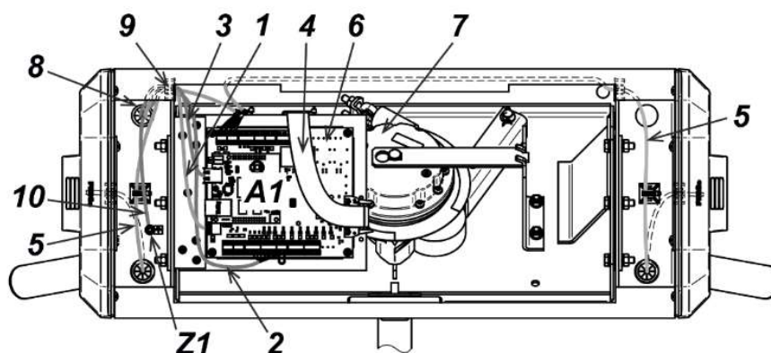
Рисунок 14. Схема прокладки кабелей в стойке ЭП
