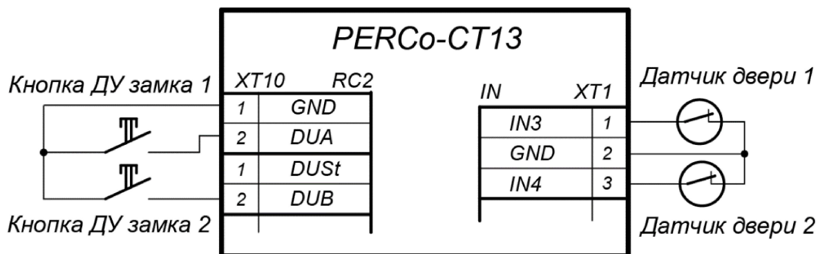
Рисунок 17. Схема подключений кнопок ДУ и датчиков двери
