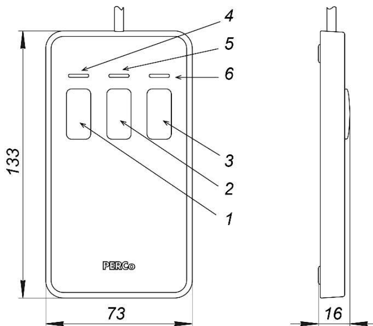
Рисунок 7. Общий вид и габаритные размеры ПДУ
