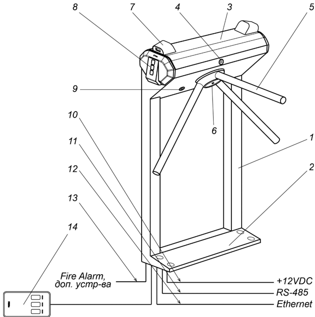
Рисунок 2. Устройство ЭП
