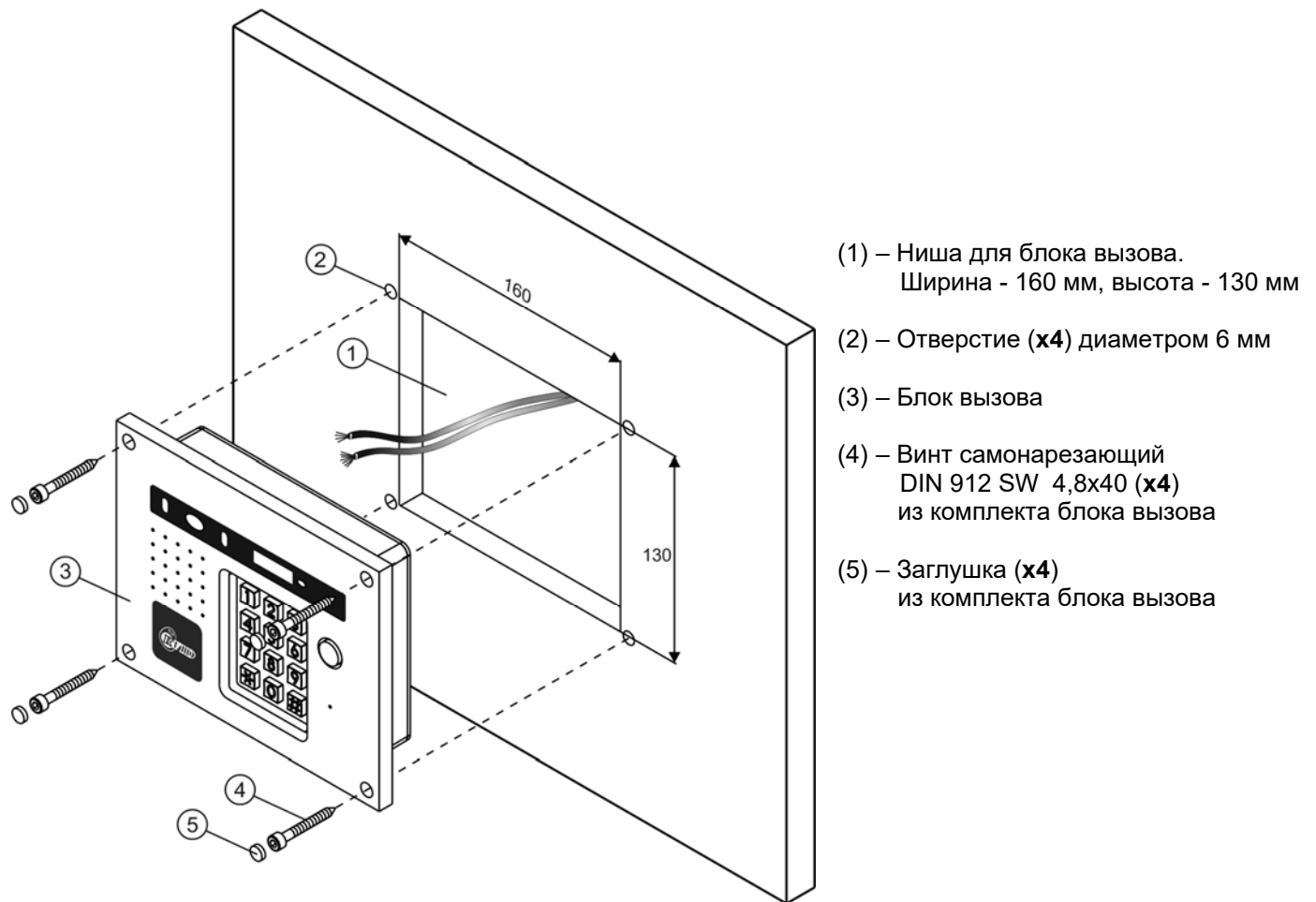
Рисунок 6.2 - Установка блока вызова на неподвижной части металлической двери
