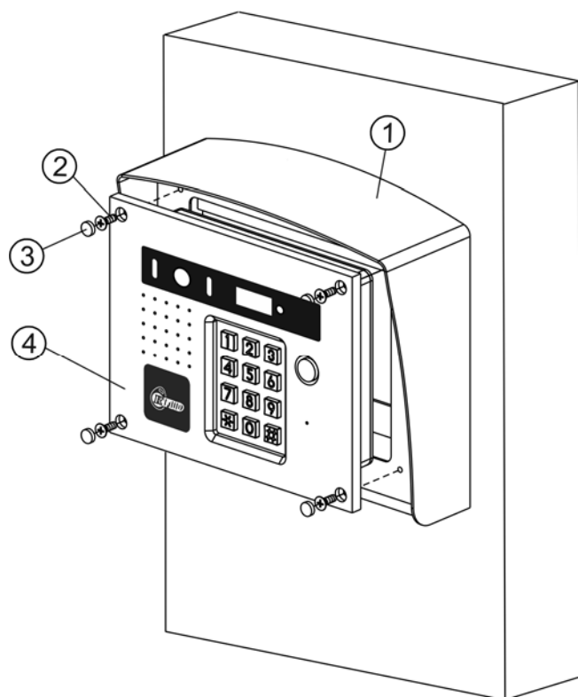
Рисунок 6.4 - Установки блока на монтажный комплект МКФ-432
