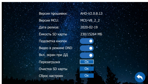
Рис. 25 Подменю "Управление"
