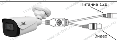
Рис.1 Схема подключения
