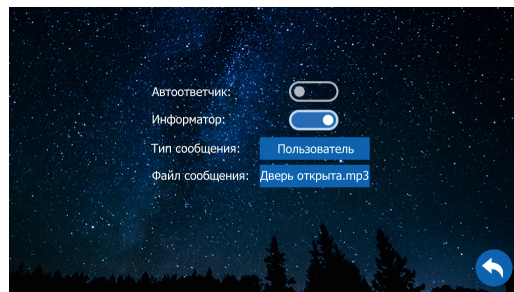
Рис. 24 Подменю "Сообщения"
