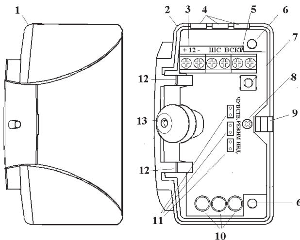
Рисунок 2 - Конструкция извещателя
