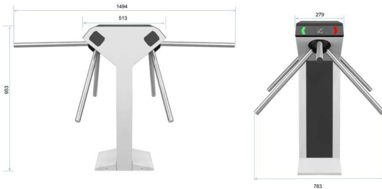
Рисунок 5.1 - Габаритные размеры турникета с планками «STR-04»
