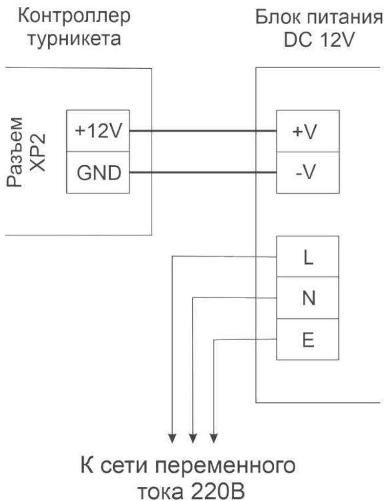
Рисунок 8.4.1 - Подключение питания к турникету
