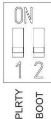
Рисунок 6.3.1 Контроллер управления турникетом «CBU-240» Dip-переключатели
