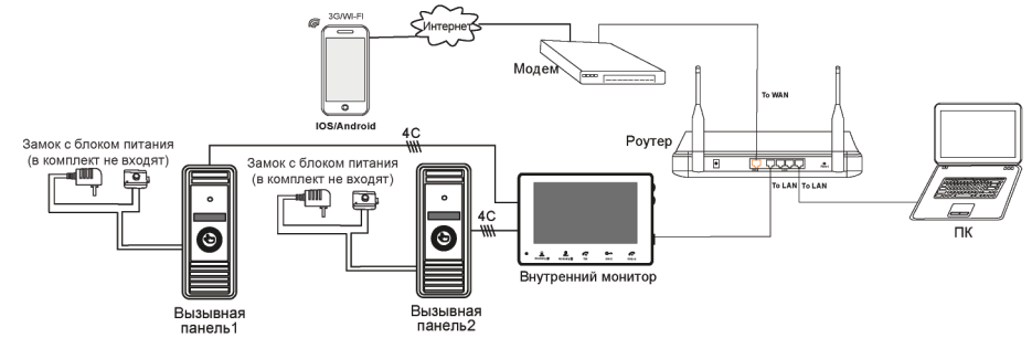
Рис. 1 – проводная схема подключения к сети.
