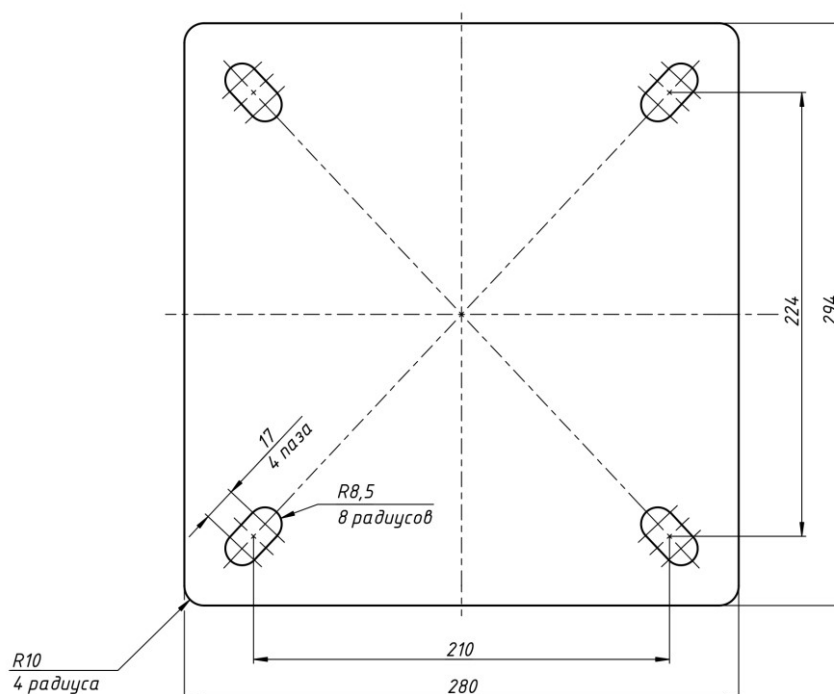
Рисунок 6.4.2 Монтажное основание
