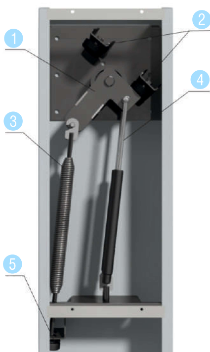
Рисунок 5.1 Устройство шлагбаума
