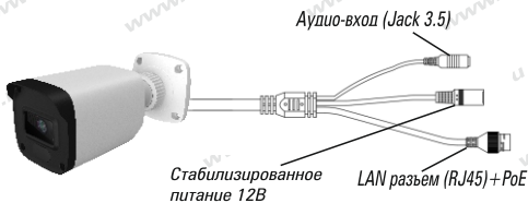
Рис. 1 Схема подключения
