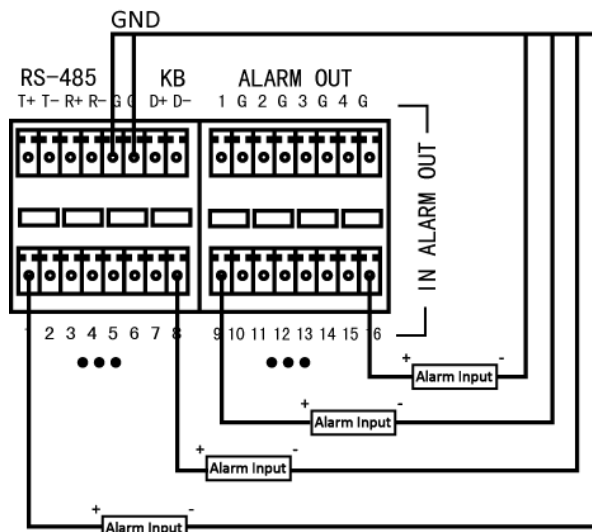
Рис. 2.5. Схема подключения тревожных входов
