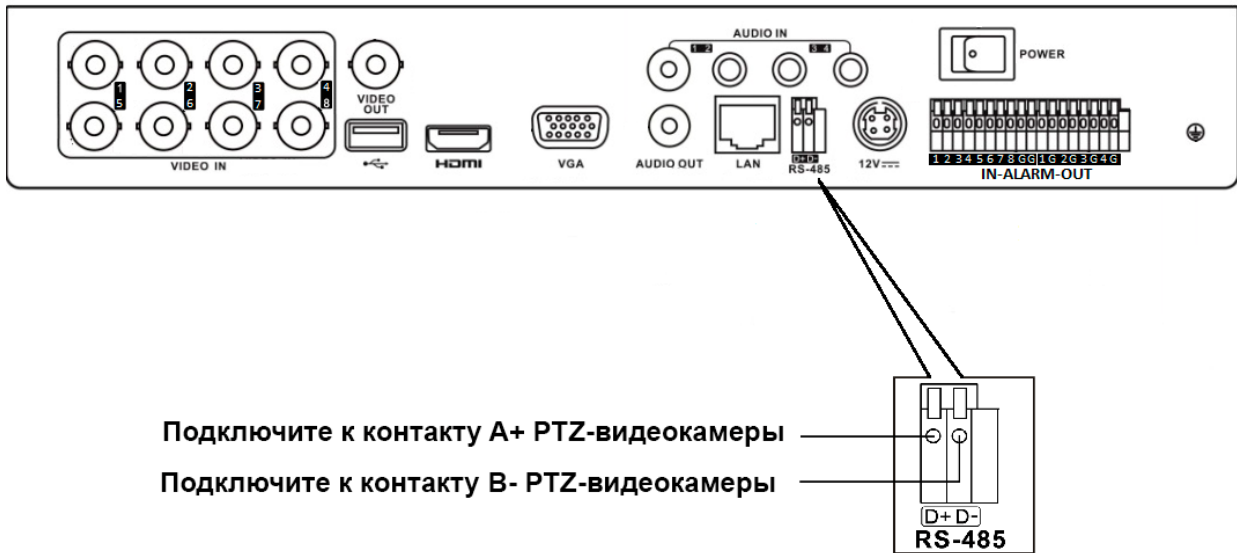
Рис. 2.4. Подключение PTZ-видеокамеры
