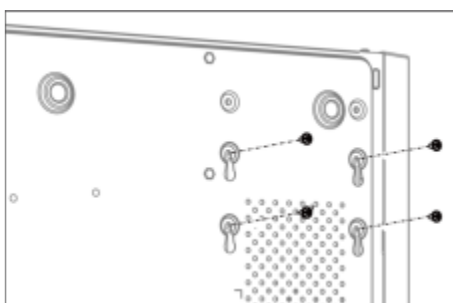
Рис. 2.3. Крепление диска
