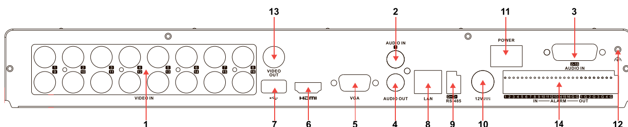
Рис. 1.4. Задняя панель видеорегистраторов LTV RTP-160 00
