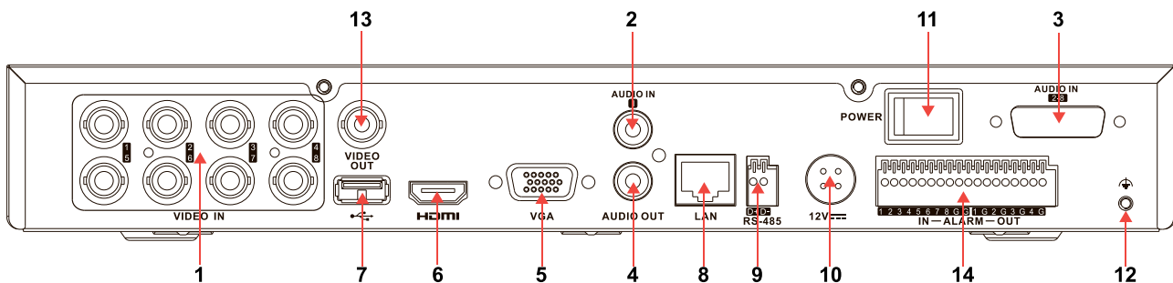
Рис. 1.3. Задняя панель видеорегистраторов LTV RTP-080 00
