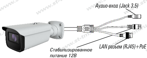
Рис. 1 Схема подключения
