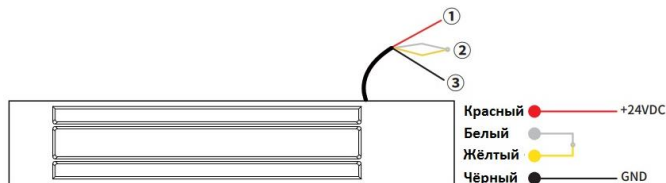
Подключение 24В
