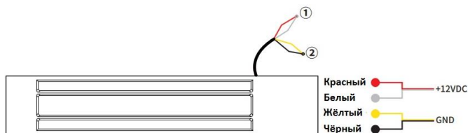
Подключение 12В
