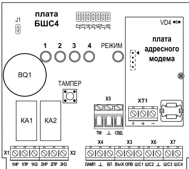
Рис.10 Плата БШС4
