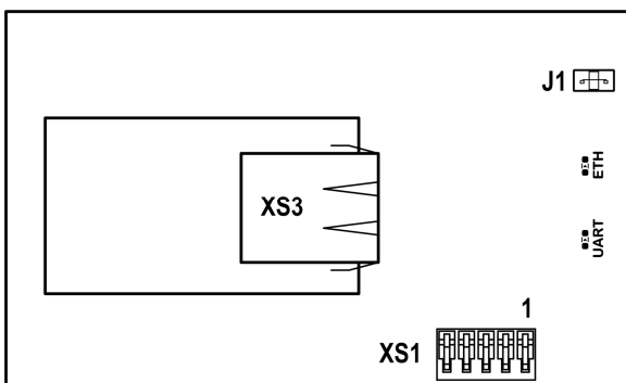
Рис. А18 Внешний вид платы IP-коммуникатора
