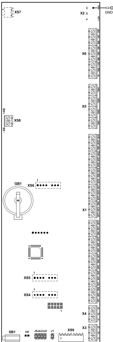
Рис.2 Плата контроллера ЦБ
