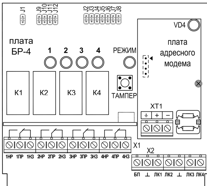
Рис.14 Плата БР-4
