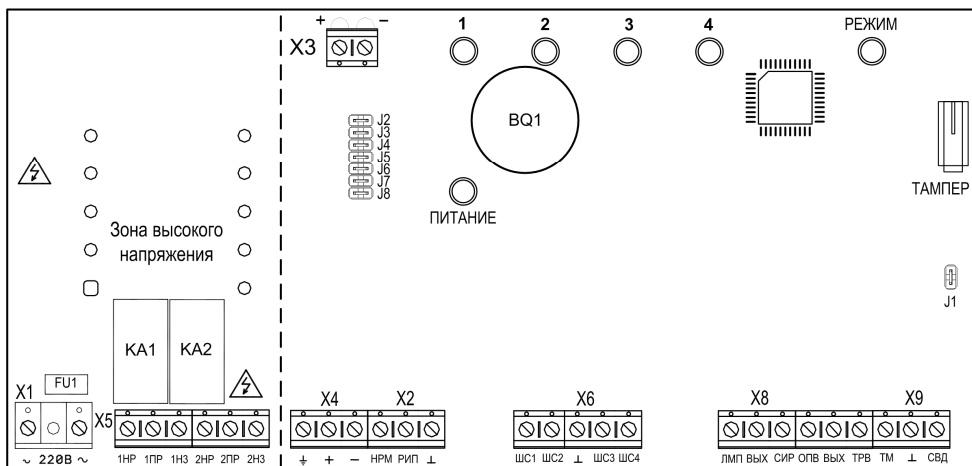
Рис. 12 Плата БШС4П
