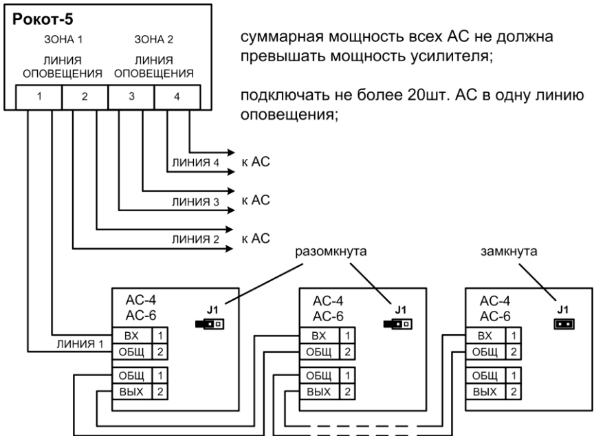
Рис.5а Схема подключений АС-4, АС-6 к линиям оповещения
