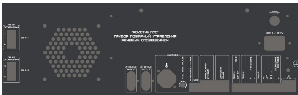
Рис.3 Внешний вид задней панели прибора
