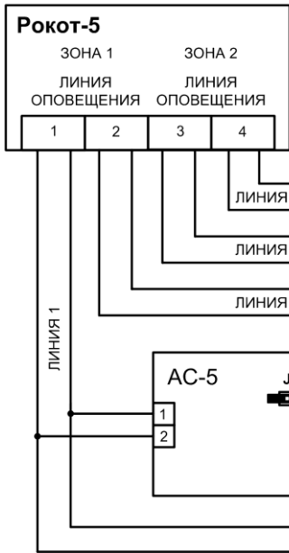
Рис.5б Схема подключений АС-5 к линиям оповещения
