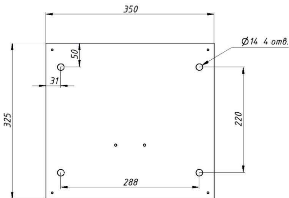
Монтажное основание
