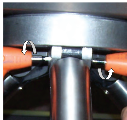
3. Затяните винты (шестигранник 5 мм)
