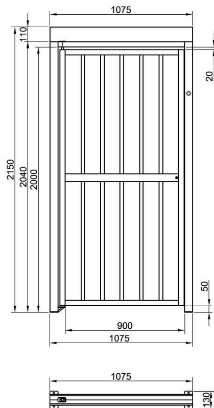
КАЛИТКА ПОЛНОРОСТОВАЯ GUARDIAN GATE 001PSSGS - Калитка электромеханическая.
