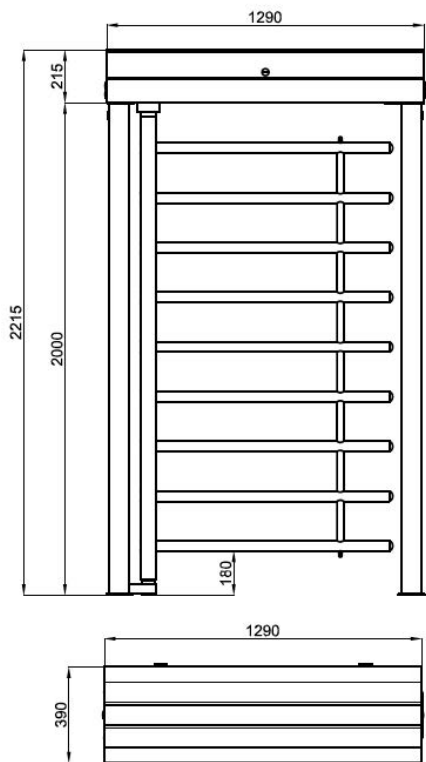
КАЛИТКА ПОЛНОРОСТОВАЯ GUARDIAN GATE BTX 100 001PSSGSA - Калитка моторизованная.
