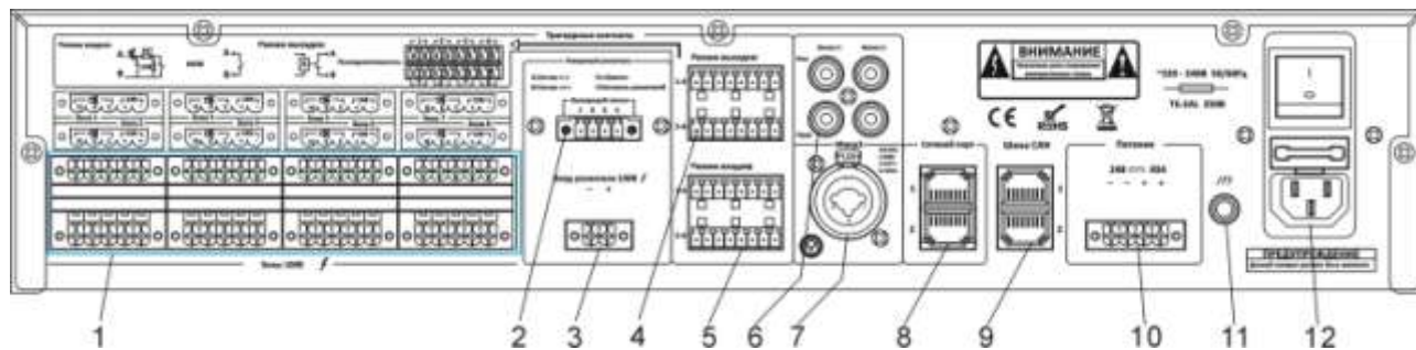
Рис. 3.3. Задняя панель усилителя мощности LPA-EVA-8500
