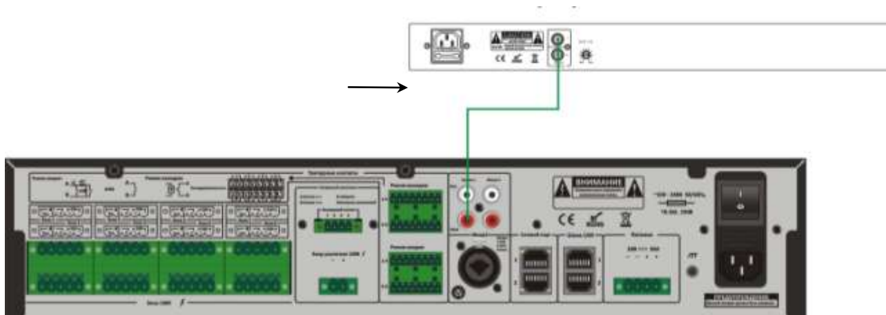
Рис. 4.1. Схема подключения источника аудиосигнала к линейным входам усилителя мощности LPA-EVA-8500
