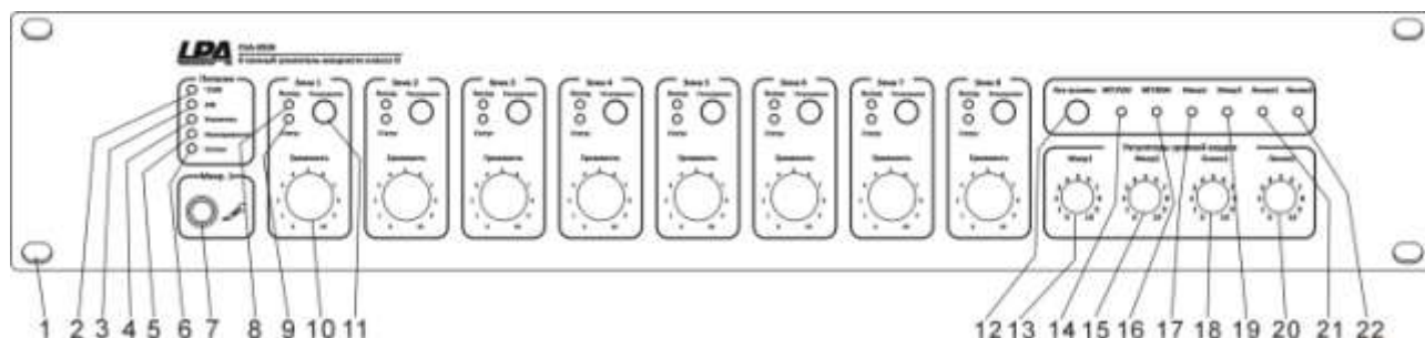
Рис. 3.2. Лицевая панель усилителя мощности LPA-EVA-8500
