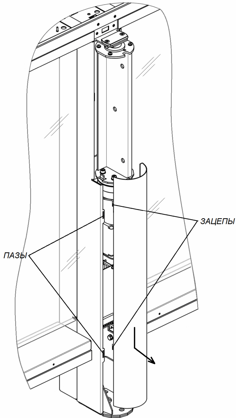
Рисунок 18. Снятие кожуха центральной стойки
