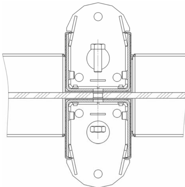
Рисунок 25. Крепление стекла заполнения в центральной стойке двусторонней секции PERCo-STD-01
