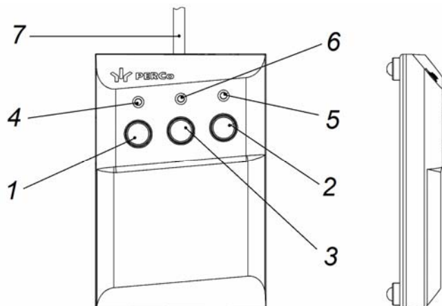
Рисунок 7. Общий вид и габаритные размеры ПДУ
