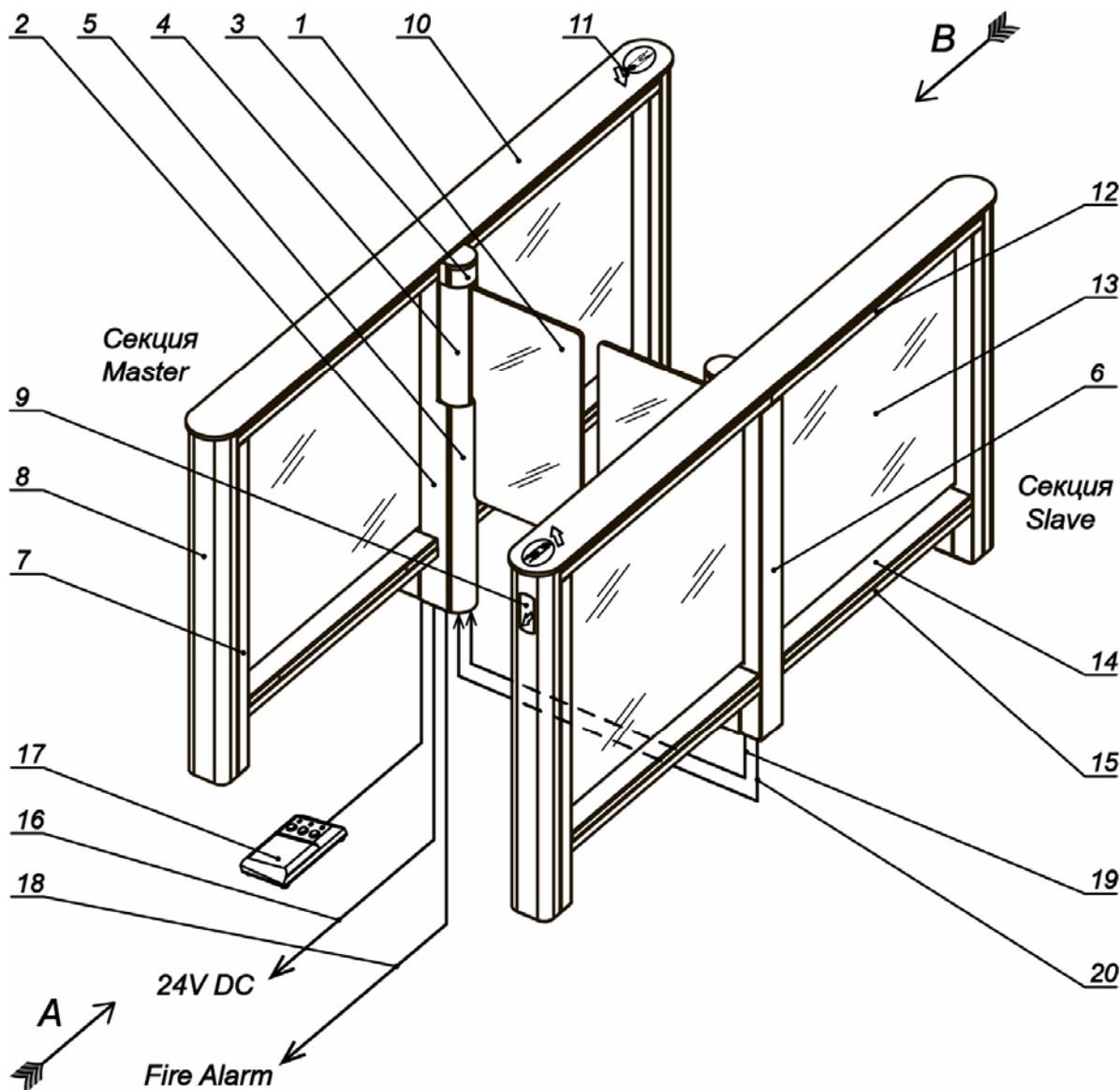
Рисунок 5. Внешний вид и устройство PERCo-ST-01:
