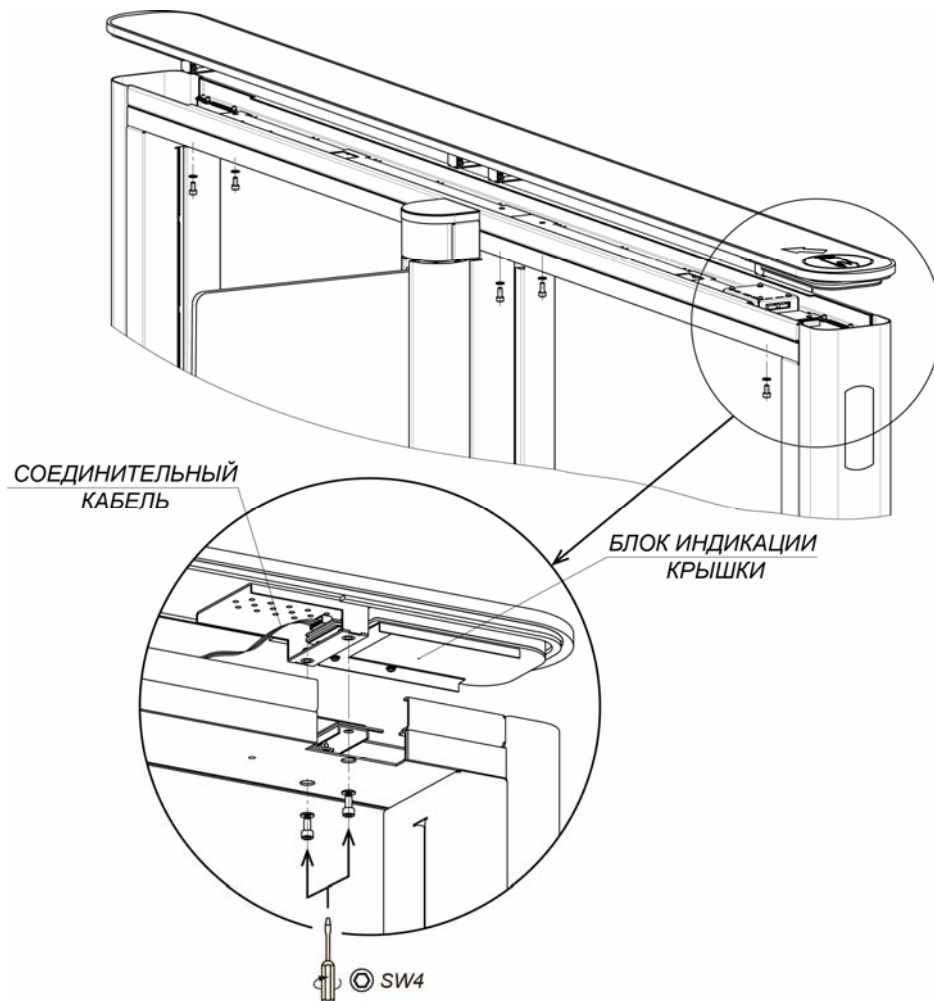
Рисунок 22. Установка крышки секции
