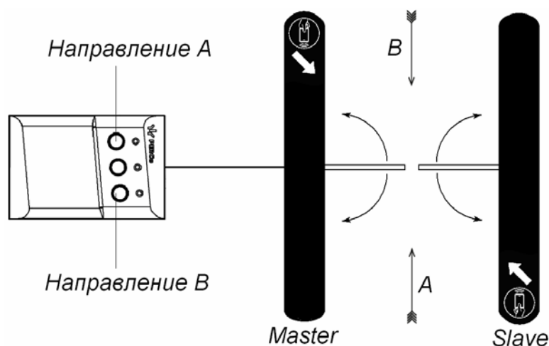
Рисунок 11. Стандартная ориентация ПДУ относительно секций турникета
