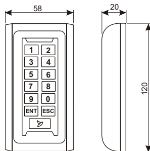
Рис.1 Габариты считывателя
