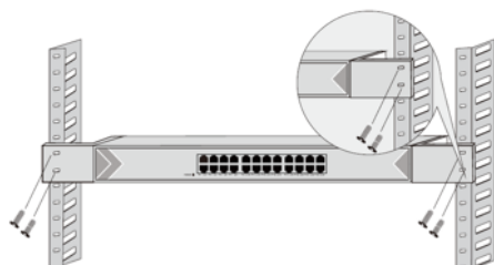
Рисунок 2.7 Установка коммутатора в стойку
