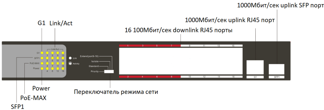
Рисунок 1.7 DS-S1816P
