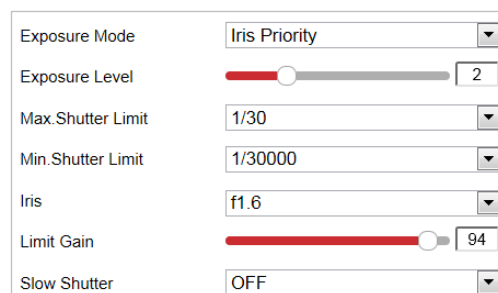
Рисунок 6-25 Настройка диафрагмы вручную
