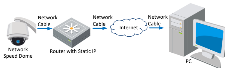
Рисунок 2-10 Доступ к IP-камере через роутер со статическим IP-адресом
