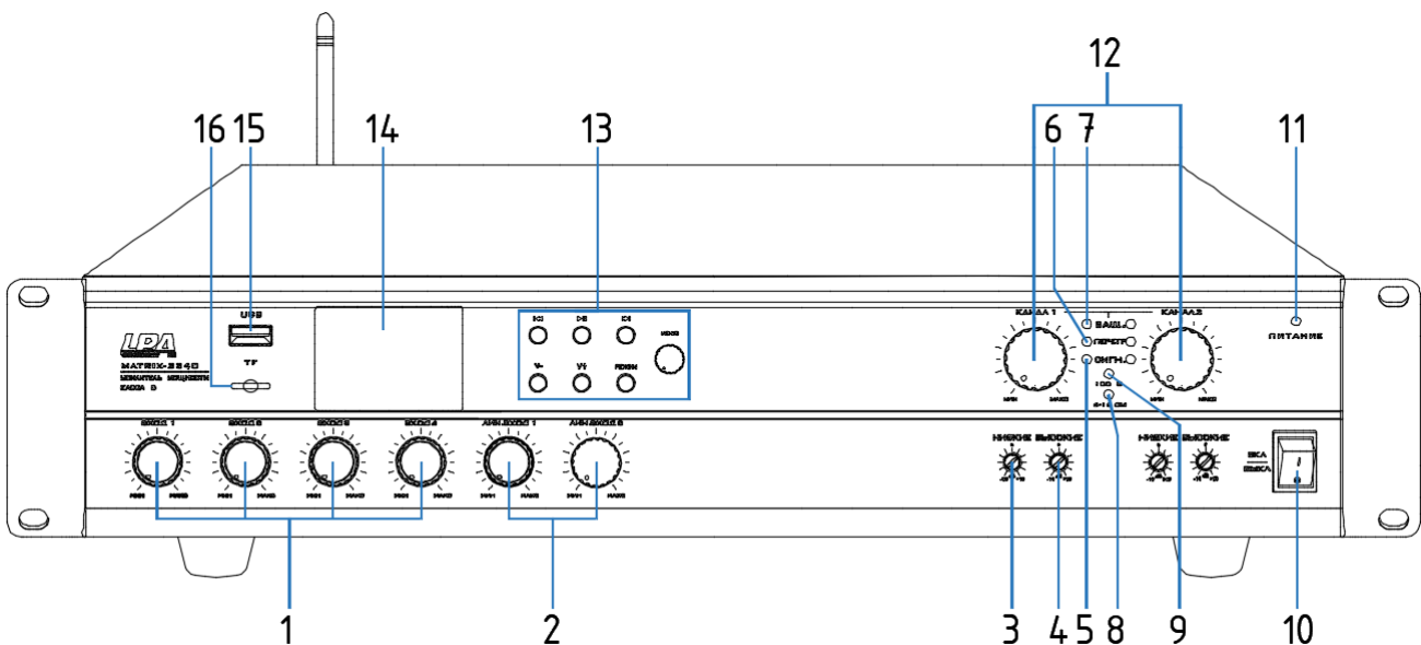
Рис.2.2. передняя панель
