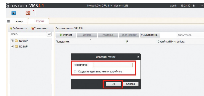
Рис. 42 Создание группы
