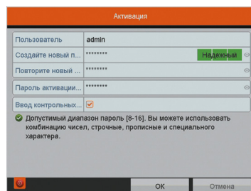
Рис. 11 Активация видеорегастратора
