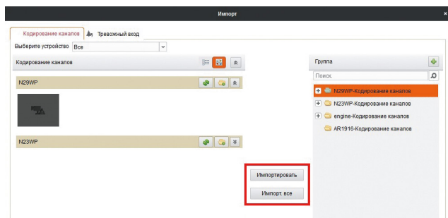
Рис. 44 Окно импорта
