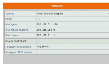
Рис. 17 Настройка сети
