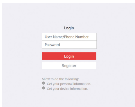
Рис. 40 Окно авторизации
