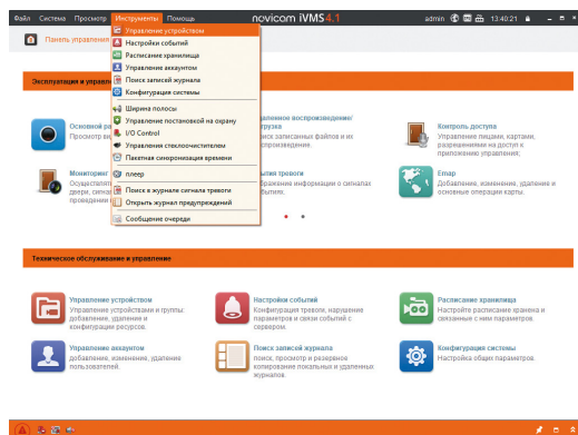
Рис. 36 Управление устройством
