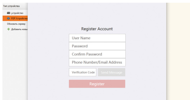
Рис. 39 Регистрация аккаунта
