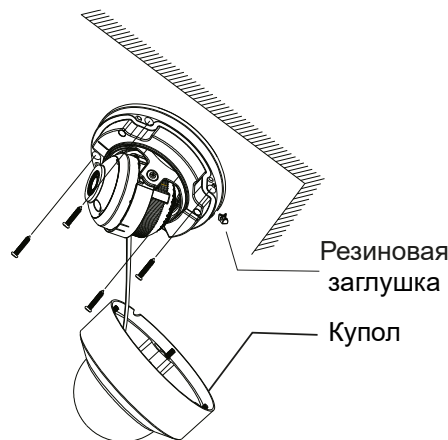
Рис. 5.2. Крепление к поверхности
