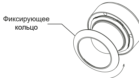
Рис. 5.1. Снятие фиксирующего кольца
