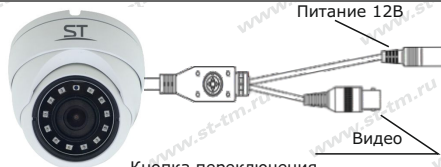
Рис.1 Схема подключения
