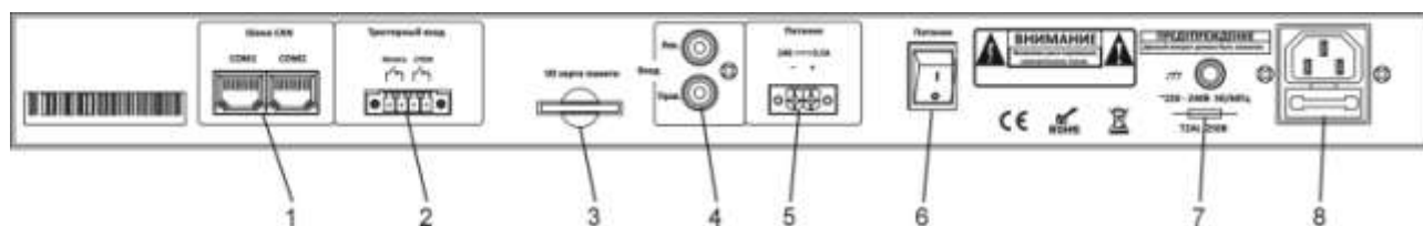
Рис. 3.3. Задняя панель блока записи сообщений LPA-EVA-RC
