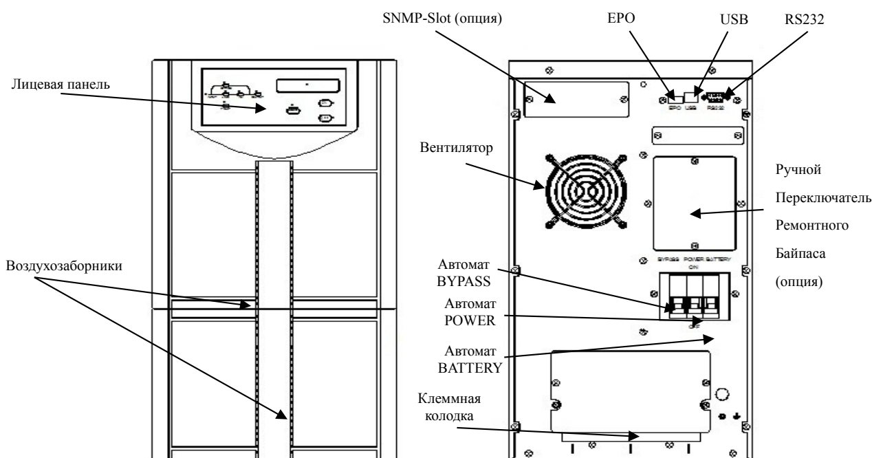
Рис.3.3-3 Внешний вид ИБП INELT серии Monolith K 6k-10k
